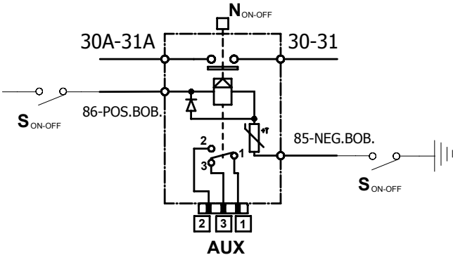
Fig. 1: Schema elettrico
