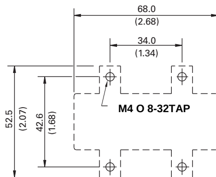
DETALLE DEL MONTAJE
