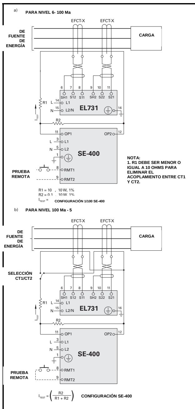
FIGURA 10: circuito de prueba de falta a tierra
