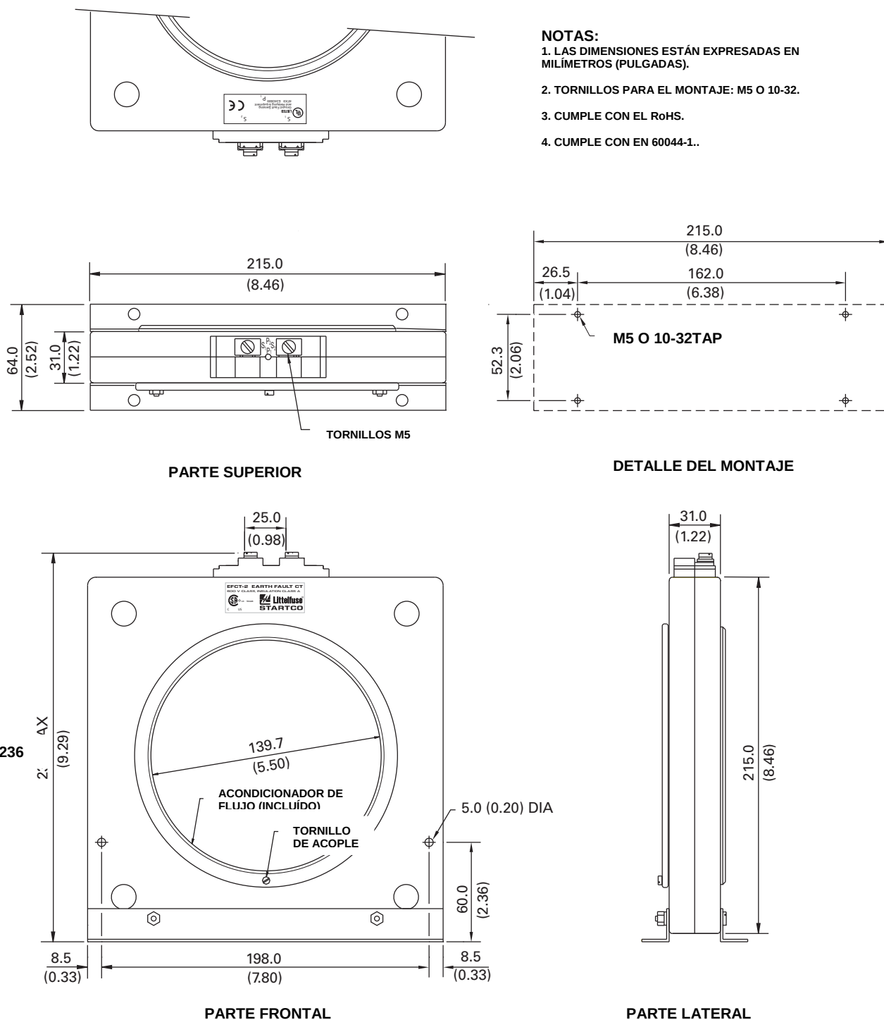
FIGURA 8. Esquema y detalles de montaje del EFCT-2
