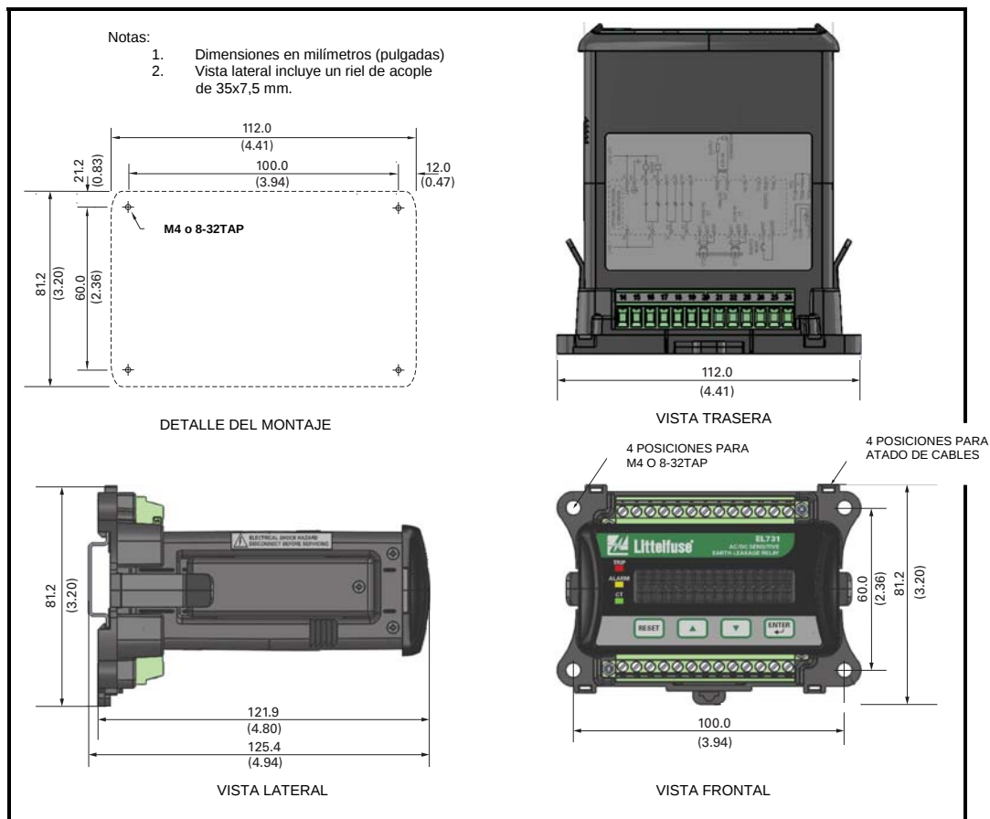
FIGURA 2. Esquema y detalles de montaje del AC700-SMK
