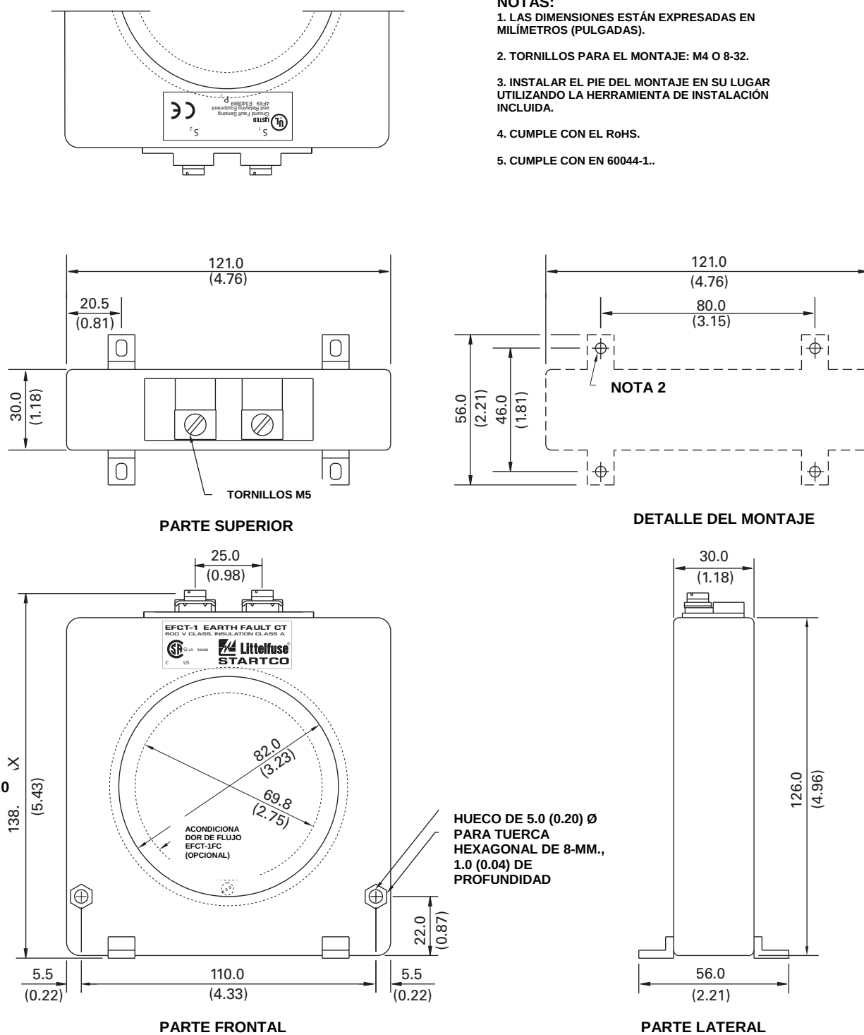
FIGURA 7. Esquema y detalles de montaje del EFCT-1
