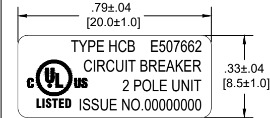
UL LABEL
