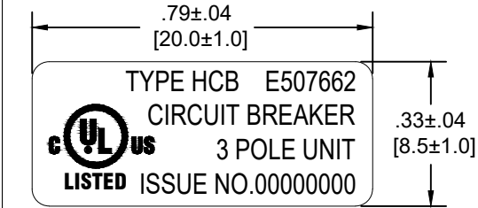
UL LABEL
