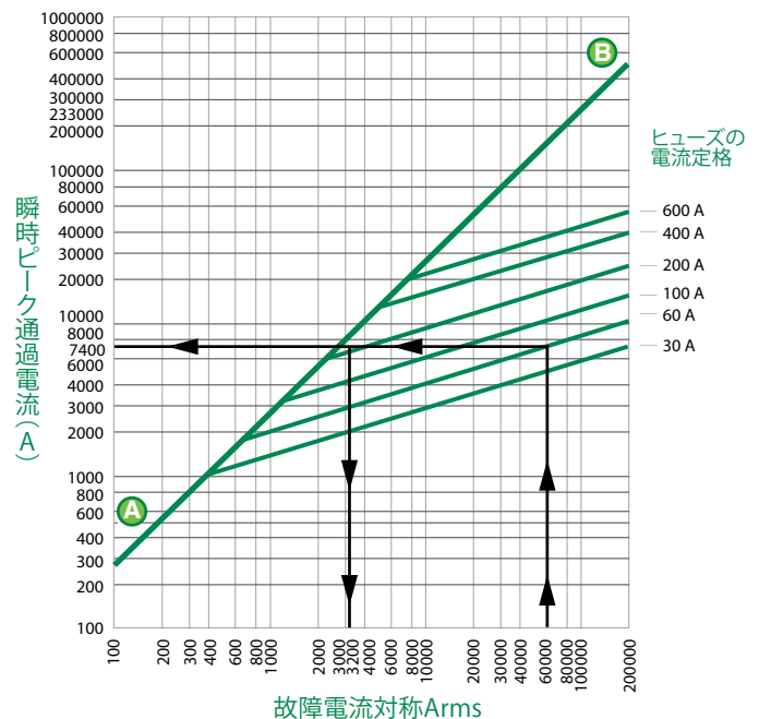
図4. リテルヒューズJTD_IDクラスJヒューズのピーク通過曲線
