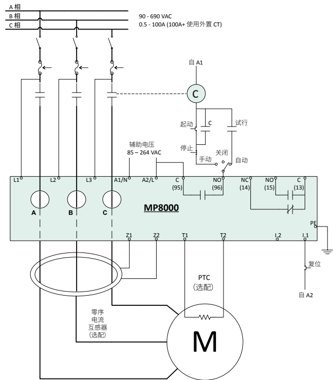
典型三相系统的接线图
