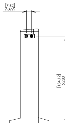
側面図
