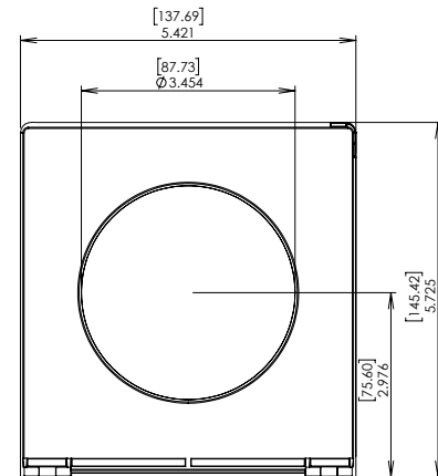
正面図
