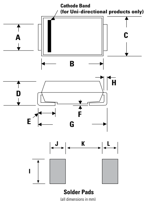
DO-214AA (SMB J-Bend)
